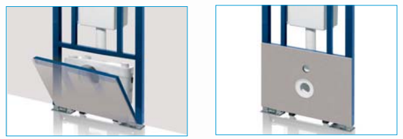
Для обеспечения доступа к насосу-измельчителю необходимо предусмотреть ревизионный люк.
